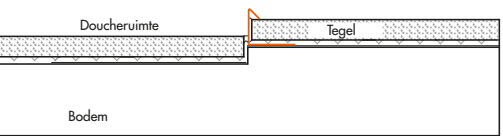
Voorbeeld 2: een dieper liggende douche met max. 16 mm niveauverschil
